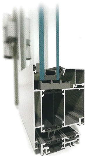
dveře MB-86 SI
