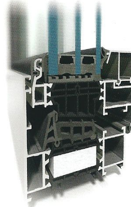
okno MB-86US Aero
