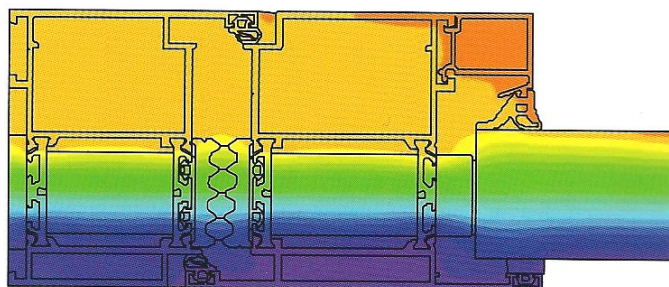
izotermický průběh ve dveřích MB-86 AERO
